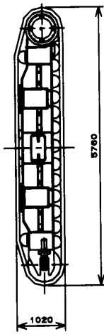
2. Side frame 7.1 ton x 2 pcs.
