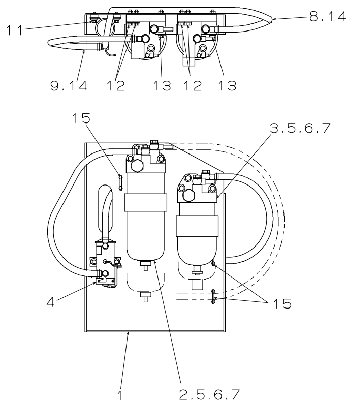
FIG.21 フューエル フィルタ セッティング FUEL FILTER SETTING
