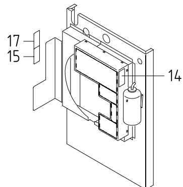
FAN SHROUD
