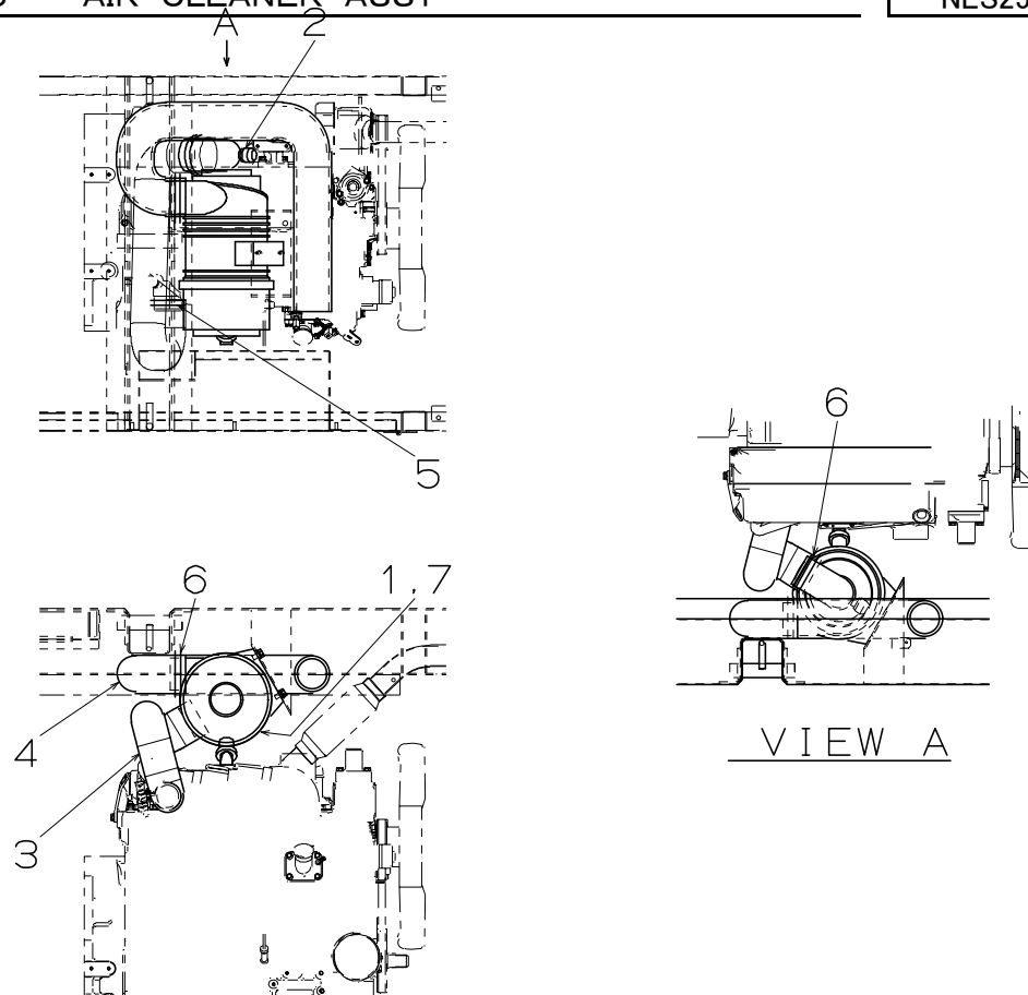
FIG.15 エア クリーナー アッセンブリ AIR CLEANER ASSY
