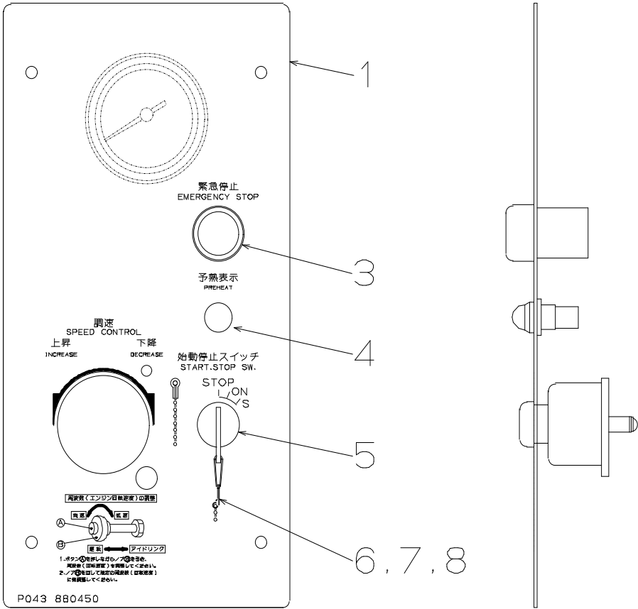
FIG.7 コントロール パネル L. アッセンブリ CONTROL PANEL L. ASSY
