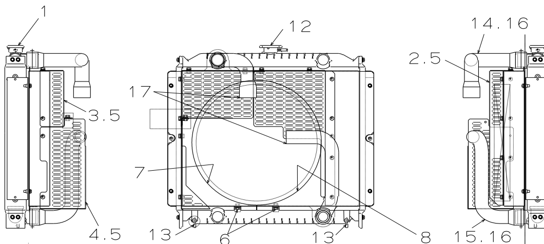
ラジエータ アッセンブリ FIG.2 RADIATOR ASSY
