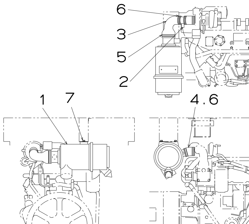
FIG.21 エアクリーナ セッティング AIR CLEANER SETTING
