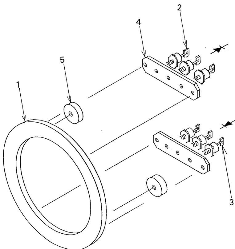
レクティファイヤ アッセンブリ FIG.4 RECTIFIER ASSY
