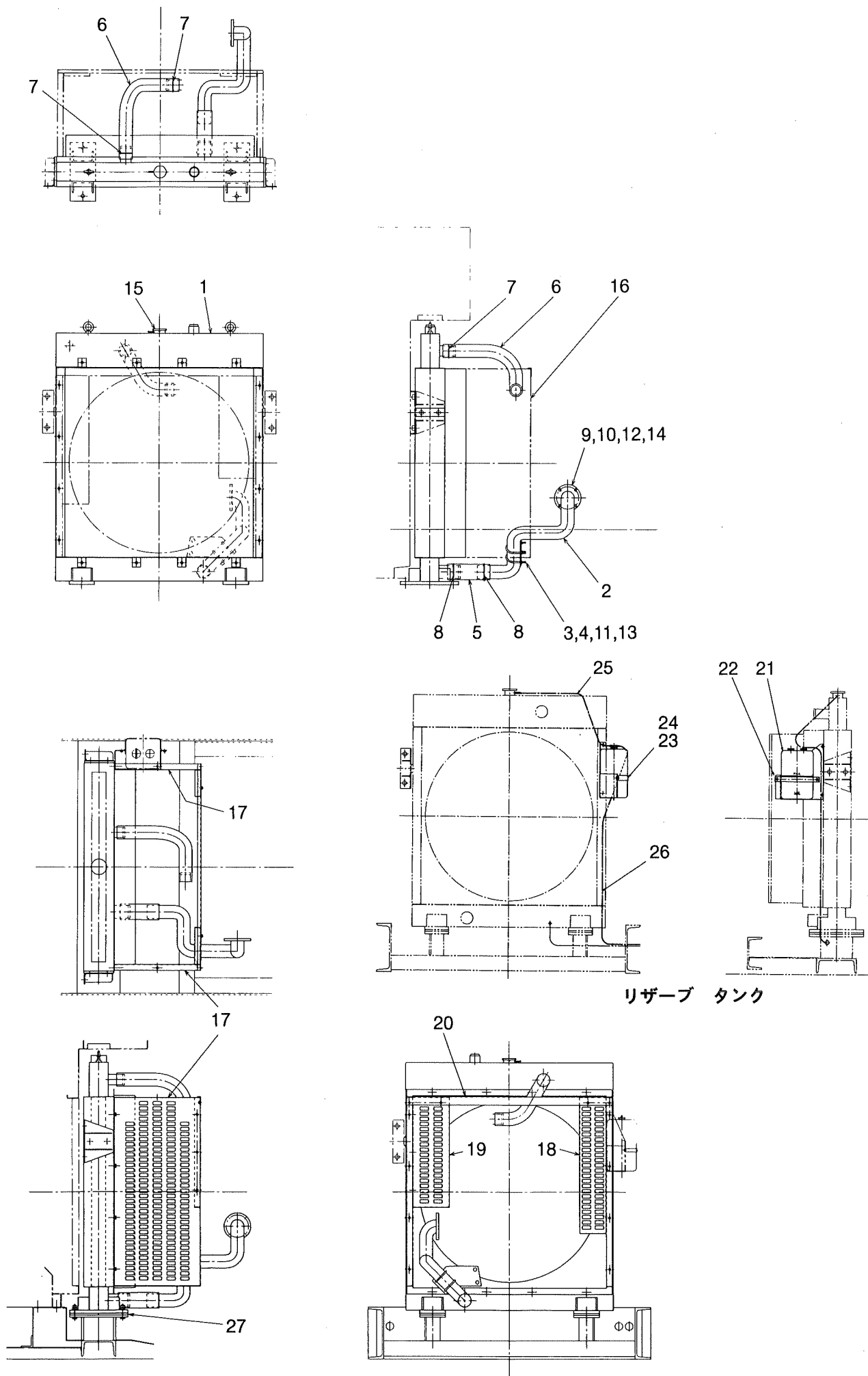
ラジエータ パイピング FIG. 2 RADIATOR PIPING
