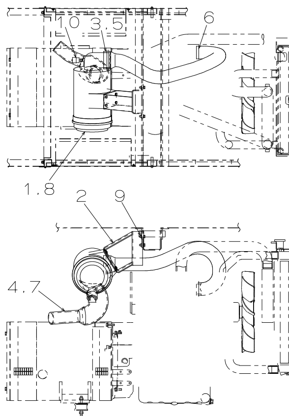
FIG.16 エアー クリーナ アッセンブリ AIR CLEANER ASSY
