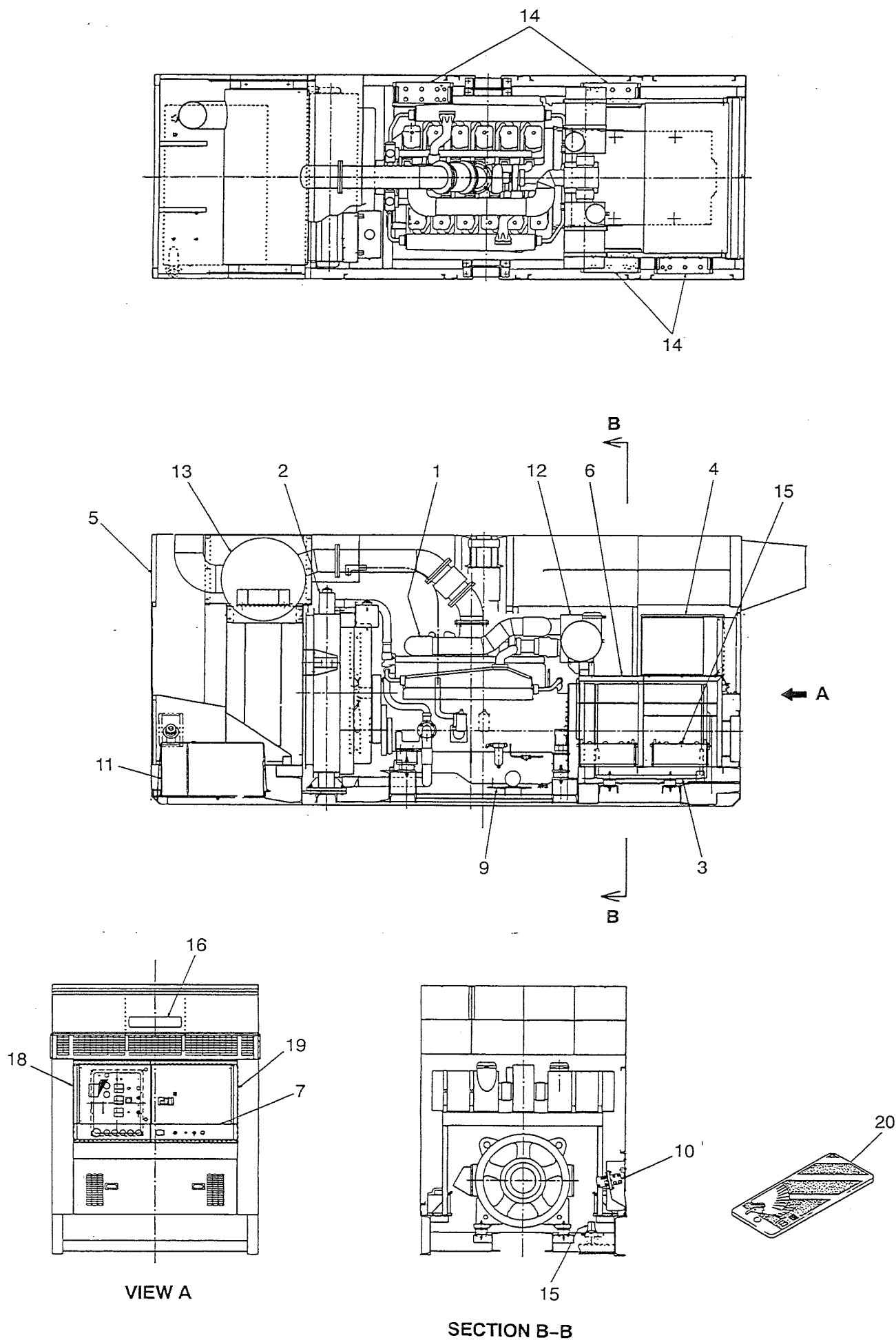
ディーゼル ジェネレータ セット FIG.1 DIESEL GENERATOR SET
